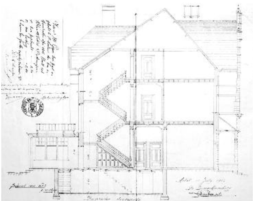
Dwarsdoorsnede
